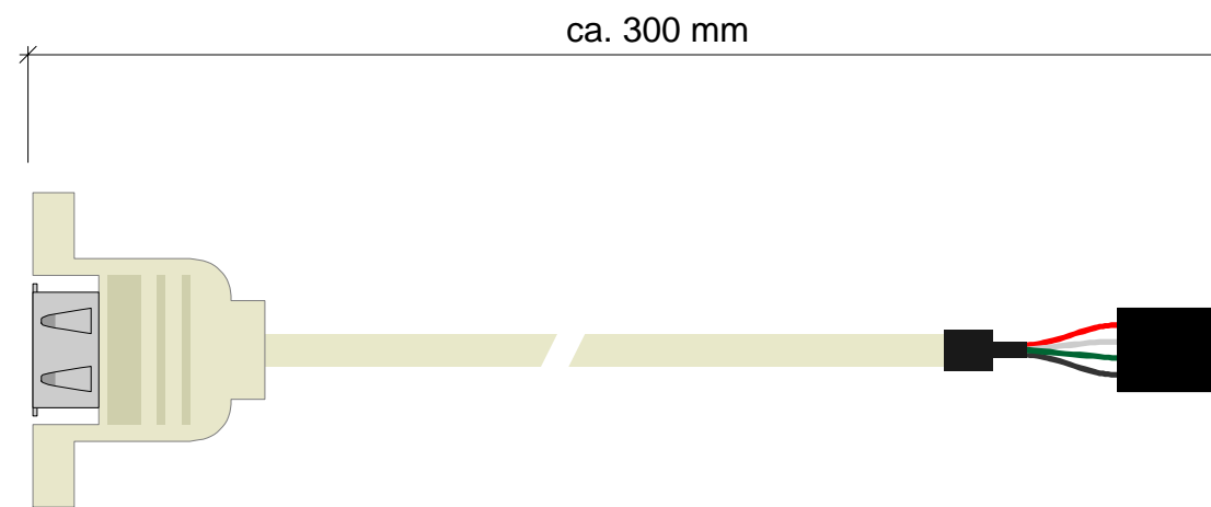
USB-Buchse auf Pfostenleiste 4 polig
